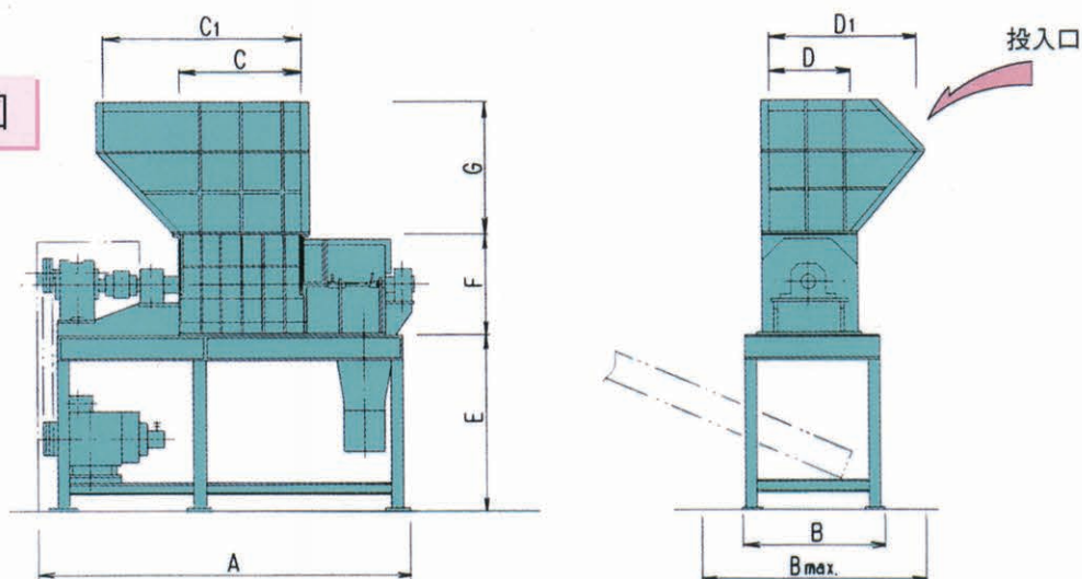
SSC-1寸法図
